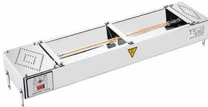
MD-90-1 尺寸 /Size: 914*150*65mm 电源功率: 220V/1000W
