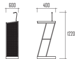
CODE : PD070003 SIZE : L600×W400×H1220mm
