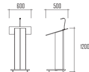
CODE : PD070001 SIZE : L600×W500×H1200mm
