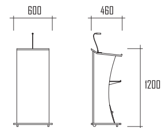
CODE : PD070002 SIZE : L600×W460×H1200mm
