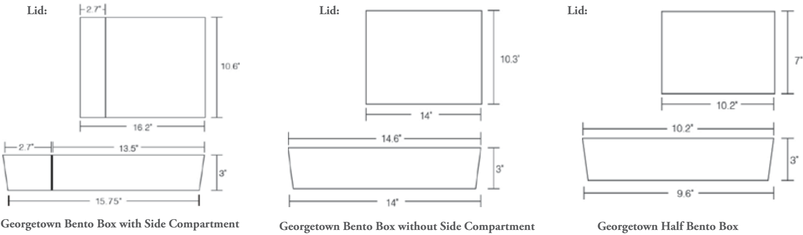
Box & Lid
